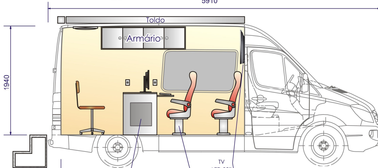
VISTA INTERNA LATERAL
