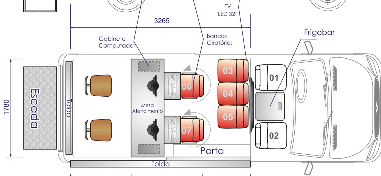
VISTA SUPERIOR
